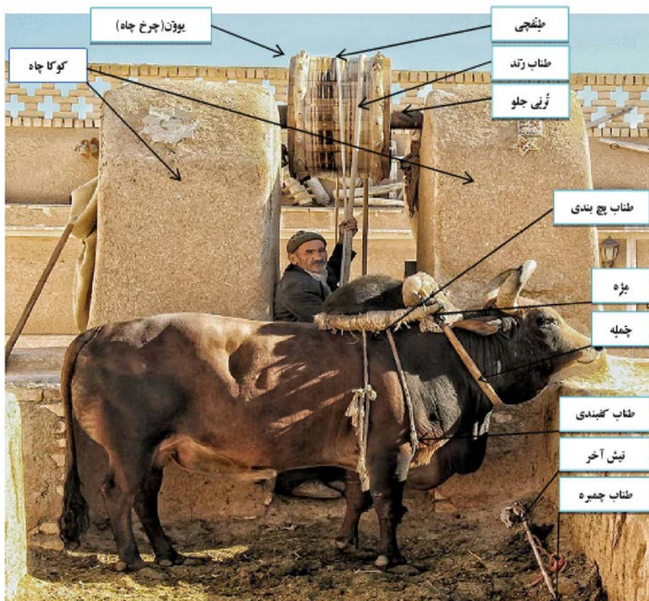
عکس ۶- اجزا و عناصر تشکیل دهنده بدنی اصلی چاه (کاکوچاه) در گاوپناه حاج ابراهیم (ورزنه)
