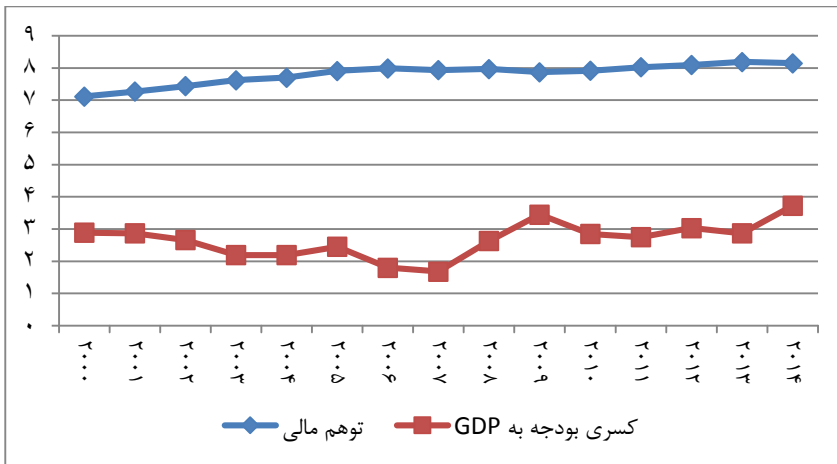
نمودار(۱): روند حرکتی میانگین توهم مالی و کسری بودجه بر GDP در کشورهای
