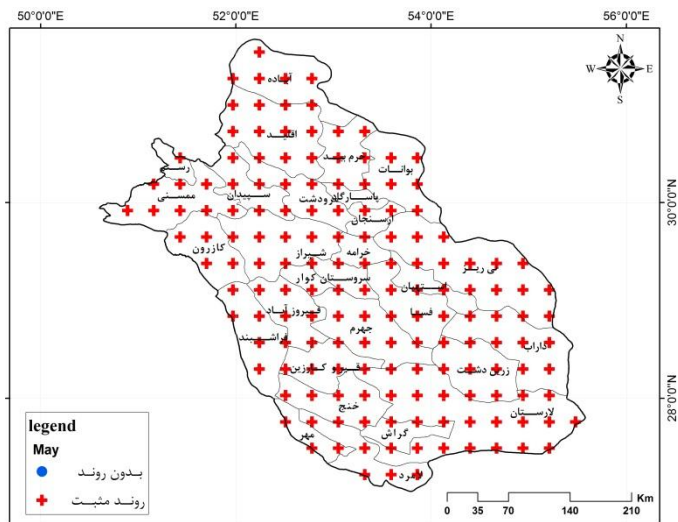
شکل ۱۱: توزیع فضایی روند درجه ساعت سرمایش می
