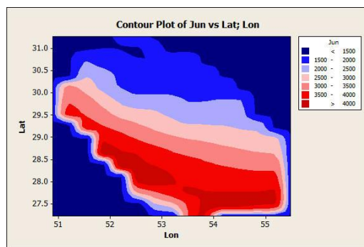
شکل ۱۹: رابطه درجه ساعت سرمایه‌ش ماهانه با عرض و طول جغرافیایی در ماه ژوئن
