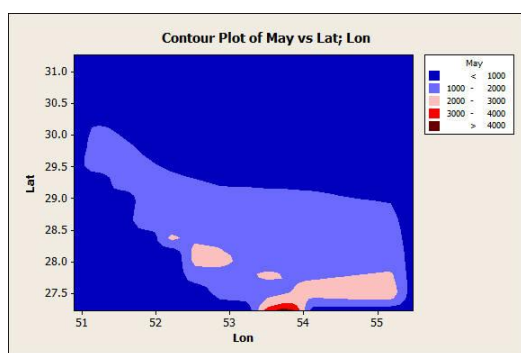
شکل ۱۸: رابطه درجه ساعت سرمایه‌ش ماهانه با عرض و طول جغرافیایی در ماه می
