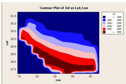
شکل ۲۰: رابطه درجه ساعت سرمایه‌ش ماهانه با عرض و طول جغرافیایی در ماه ژولای
