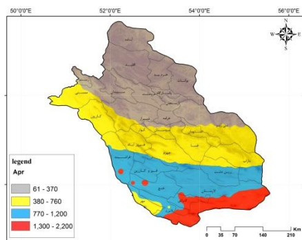
شکل ۳: جمع میانگین ماهانه درجه ساعت سرمایش آوریل
