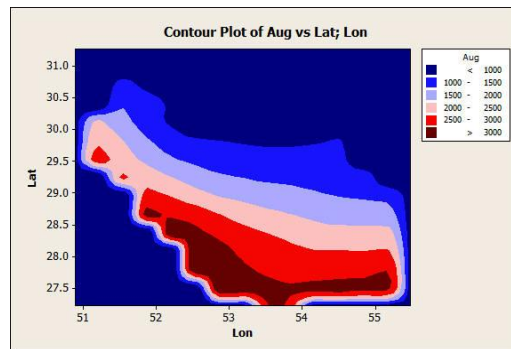
شکل ۲۱: رابطه درجه ساعت سرمایه‌ش ماهانه با عرض و طول جغرافیایی در ماه اوت
