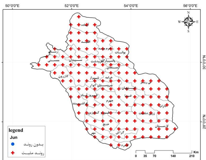
شکل ۱۲: توزیع فضایی روند درجه ساعت سرمایش ژوئن
