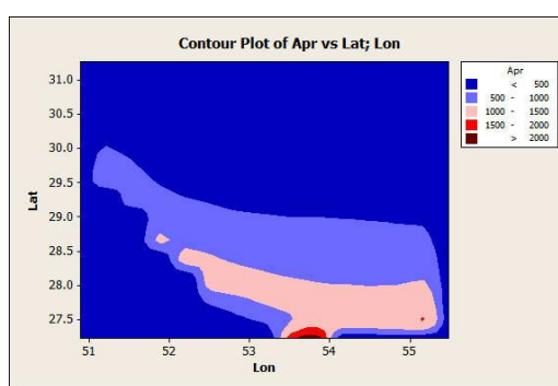
شکل ۱۷: رابطه درجه ساعت سرمایه‌ش ماهانه با عرض و طول جغرافیایی در ماه آوریل
