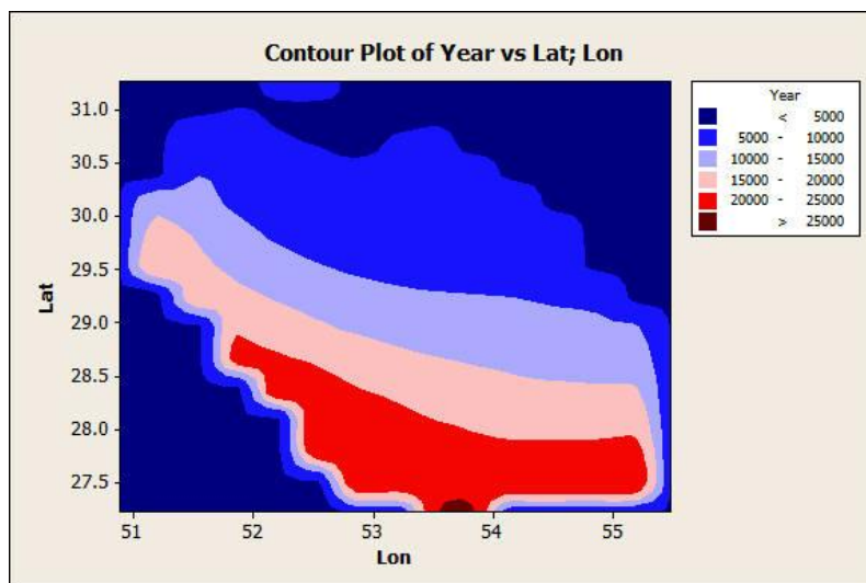
شکل ۲۳: رابطه میانگین سالانه درجه ساعت سرمایه‌ش با عرض و طول جغرافیایی
