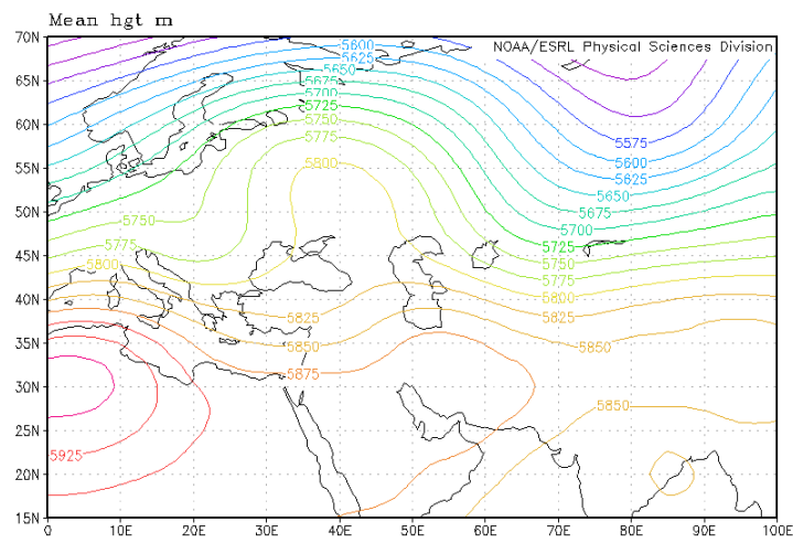
شکل ۱۰: الگوی متوسط توپوگرافی سطح ۵۰۰ هکتوپاسکال تیرماه ۱۳۸۰
