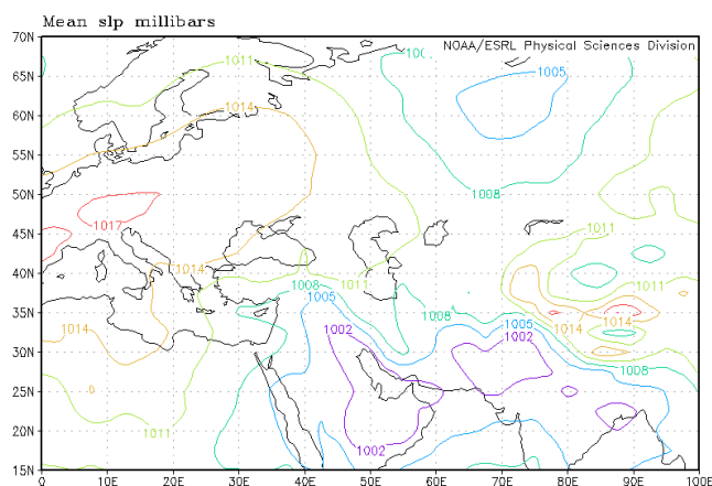
شکل ۱۲: الگوی متوسط توزیع فشار سطح دریا مرداد ۱۳۸۰
