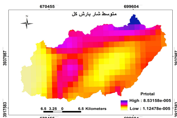
شکل ۲۴: تغییرات مکانی متوسط سالانه شار کل بارش
