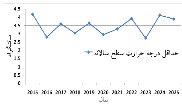
شکل ۱۹: تغییرات سالانه کمینه دما سطح خاک
