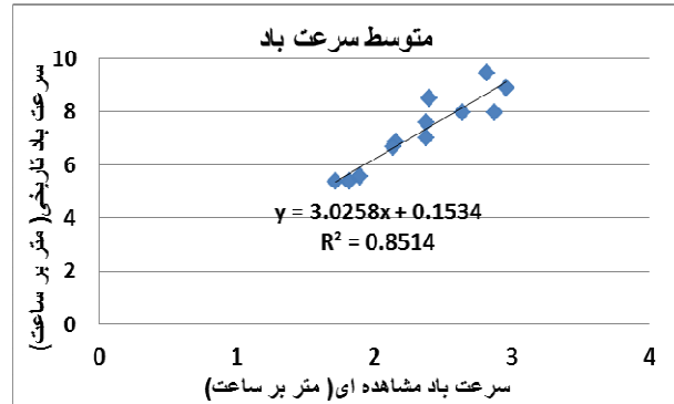
شکل ۸: متوسط سرعت باد ماهانه مشاهده‌ای و تاریخی (۲۰۰۰-۱۹۹۶).
