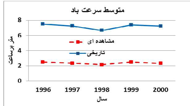
شکل ۱۲: تغییرات سالانه سرعت باد برای دوره تاریخی و مشاهده‌ای.
