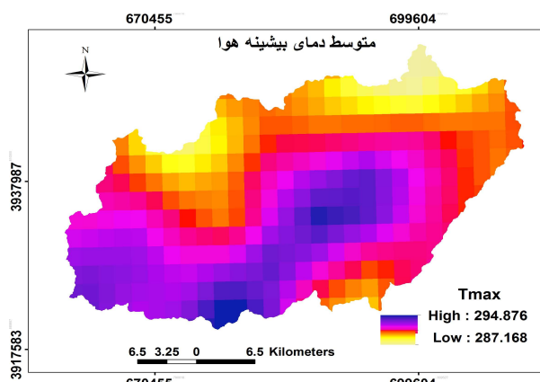
شکل ۲۳: تغییرات مکانی متوسط سالانه بیشینه دما
