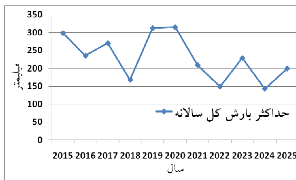
شکل ۲۰: تغییرات سالانه بیشینه بارش کل.
