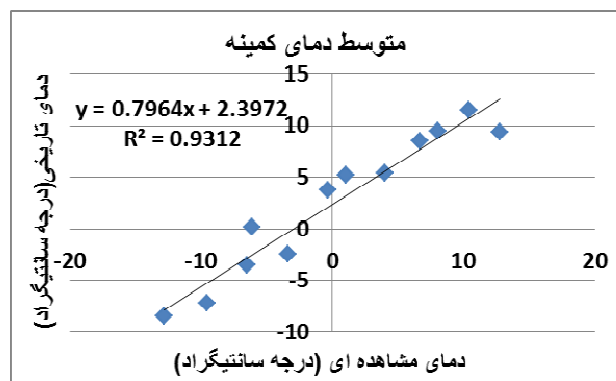
شکل ۴: رابطه متوسط دمای کمینه مشاهده‌ای و تاریخی (۲۰۰۰-۱۹۹۶).
