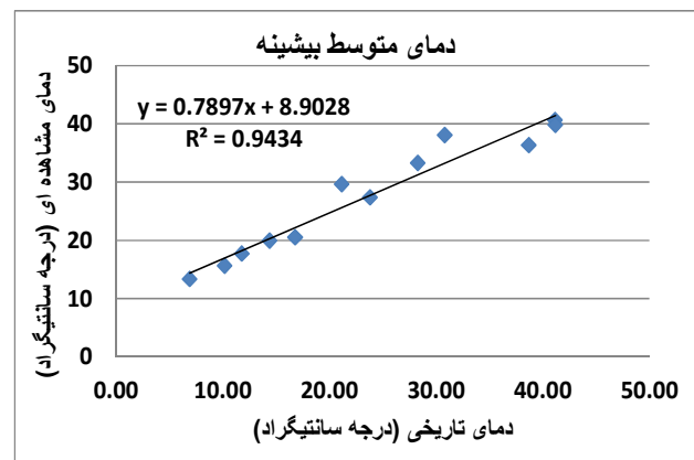
شکل ۶: رابطه متوسط دمای بیشینه ماهانه مشاهده‌ای و تاریخی (۲۰۰۰-۱۹۹۶).
