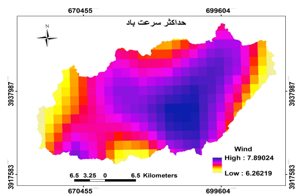
شکل ۲۵: تغییرات مکانی متوسط سالانه بیشینه سرعت باد
