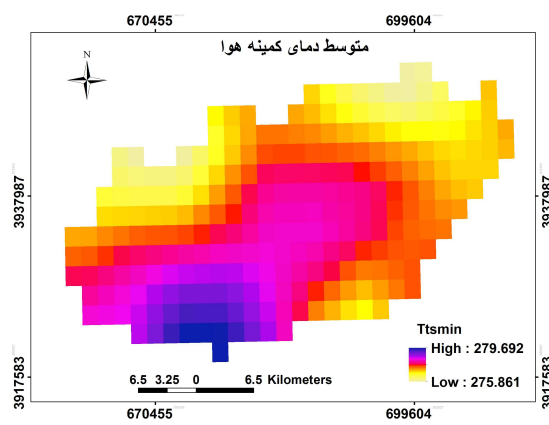
شکل ۲۲: تغییرات مکانی متوسط سالانه کمینه دما
