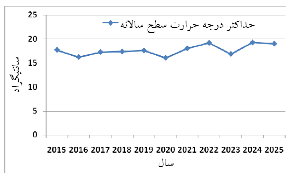
شکل ۱۸: تغییرات سالانه بیشینه دما سطح خاک.
