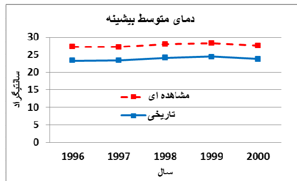
شکل ۱۰: تغییرات سالانه دمای بیشینه برای دوره تاریخی و مشاهده‌ای.
