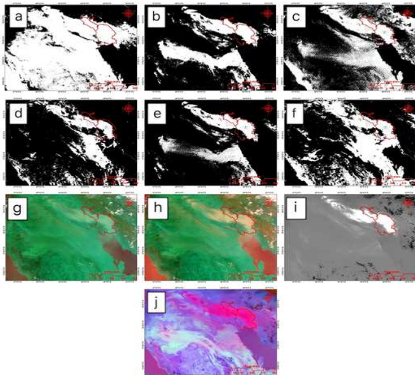
شکل ۴: خروجی روش‌های شناسایی گرد و غبار برای رویداد ۳۰ خرداد ۱۳۹۱ a و b (BTD آکرمین)، c، d، e و f (شاخص گرد و غبار)، g و h (میلر)، i (TIDI) و j (DUST RGB)
