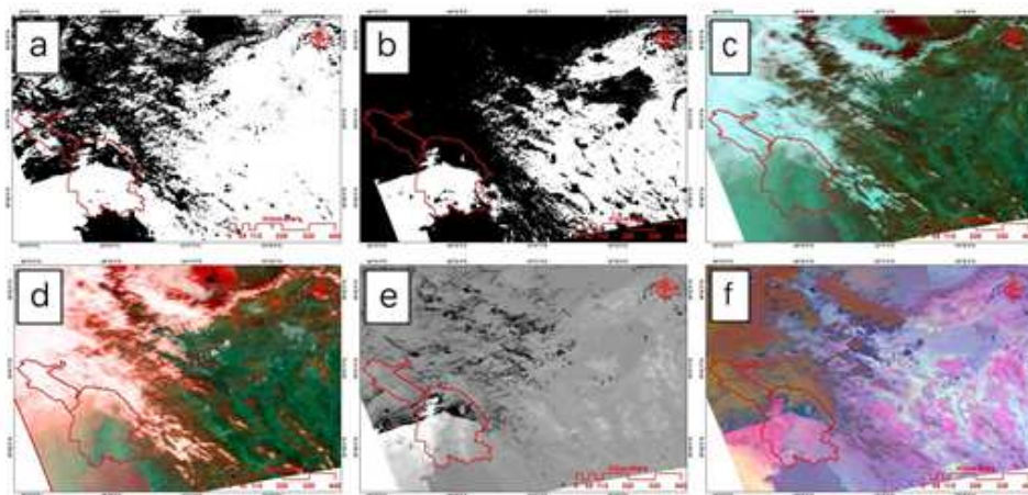
شکل ۲: خروجی روش‌های شناسایی گرد و غبار برای رویداد ۱۲ اسفند ۱۳۹۰: a و b (BTDAکرم)، c و d (میلر)، e (TIIDI) و f (DUST RGB)
