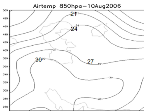
شکل ۱۷: دمای هوا ۸۵۰، ۱۳۸۵/۰۵/۱۹
