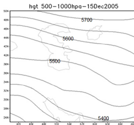
شکل ۱۱: ضخامت جو ۱۳۸۴/۰۹/۲۴
