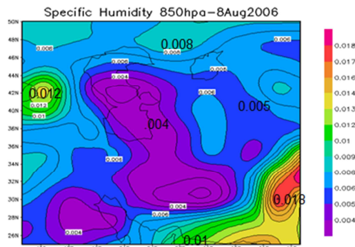
شکل ۱۸: رطوبت ویژه ۸۵۰، ۱۳۸۵/۰۵/۱۹
