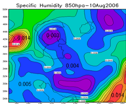
شکل ۱۹: رطوبت ویژه ۸۵۰، ۱۳۸۵/۰۵/۱۷
