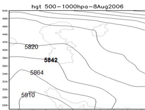
شکل ۲۱: ضخامت جو، ۱۳۸۵/۰۵/۱۹
