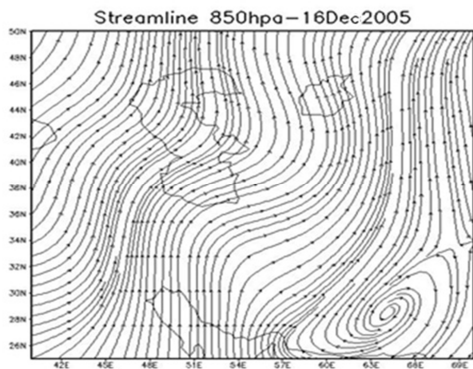
شکل ۱۴: جریان باد ۱۳۸۴/۰۹/۲۴ ۸۵۰
