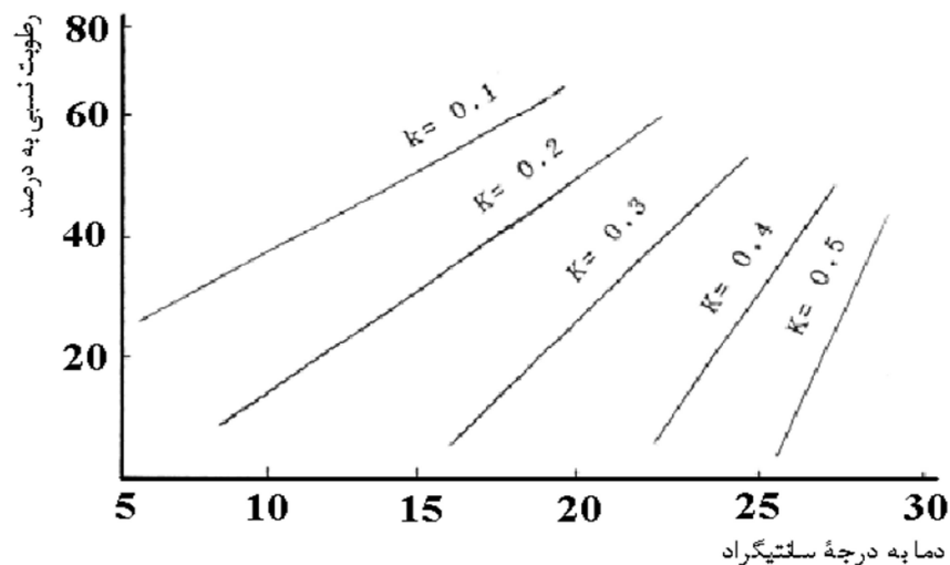
شکل ۱: نمودار ضریب خطر آتش‌سوزی فرانسیلا (شیرزادی، ۱۳۷۱ به نقل از عزیز، ۱۳۸۸)
