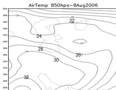
شکل ۱۶: دمای هوا ۸۵۰، ۱۳۸۵/۰۵/۱۷
