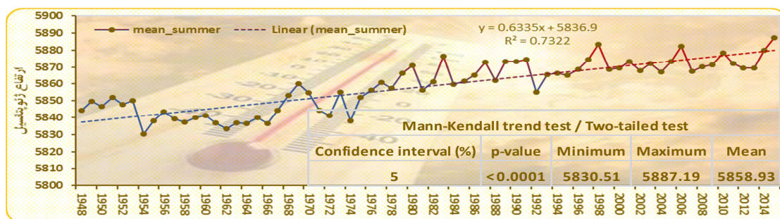
شکل ۹: روند تغییرات میانگین ۶۸ ساله ارتفاع ژئوپتانسیل نیوار ایران - فصل تابستان
