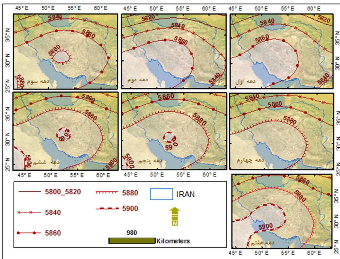
شکل ۱: شاخص سطح و شدت پرفشار جنب حاره تراز ۵۰۰ هکتوپاسکال فصل تابستان از دهه اول تا دهه هفتم
