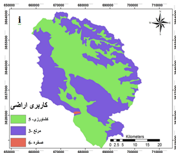
شکل ۳: فاکتورهای موثر در وقوع سیل شامل: طبقات ارتفاعی (a)، شیب (b)، انحنای زمین (c)، فاصله از رودخانه (d)، زمین‌شناسی (e)، گروه‌های هیدرولوژیک خاک (f)، نوع خاک (g)، شماره منحنی رواناب (h) و کاربری اراضی (i).
