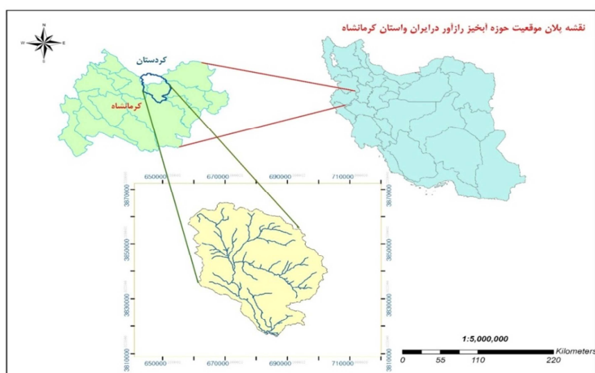
شکل ۱: نقشه موقعیت حوضه آبخیز رازآور
