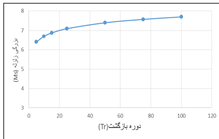
شکل ۳: نمودار بزرگی زمین لرزه و دوره بازگشت آنها
