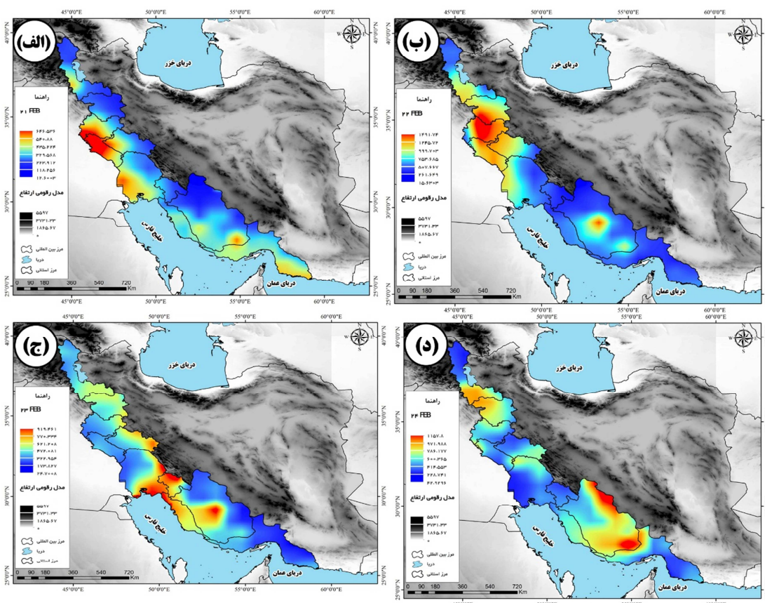
شکل ۲: توزیع فضایی ارتفاع لایه مرزی بر اساس برونداد پایگاه ECMWF نسخه ERA-Interim برای ساعت ۱۲UTC؛ (الف) ۲۱ فوریه ۲۰۱۶ میلادی؛ (ب) ۲۲ فوریه ۲۰۱۶ میلادی؛ (ج) ۲۳ فوریه ۲۰۱۶ میلادی و (د) ۲۴ فوریه ۲۰۱۶ میلادی
