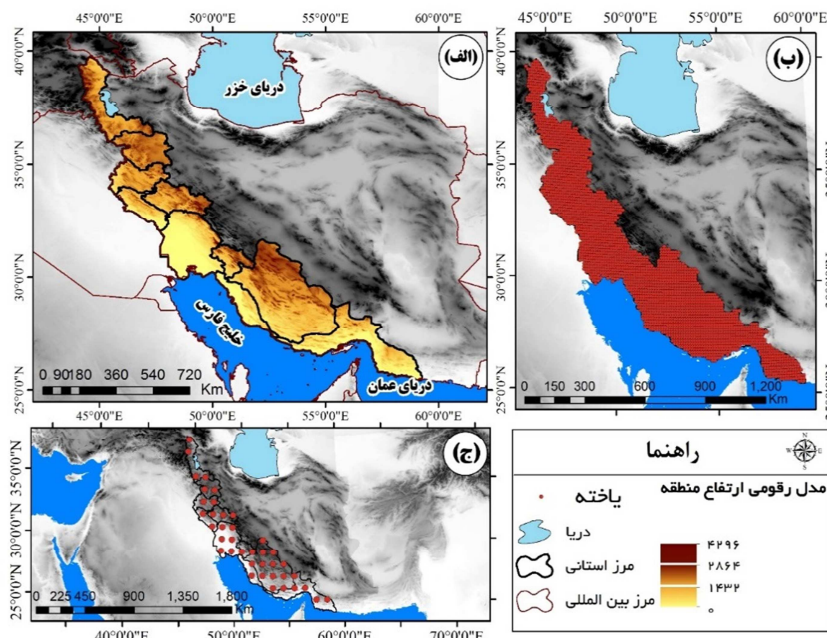
شکل ۱: منطقه مورد مطالعه؛ الف) استان‌های مورد مطالعه به همراه مدل رقومی ارتفاعی منطقه با تفکیک مکانی ۳۰ متر؛ ب) یاخته‌های جداد شده برای منطقه مورد مطالعه از پایگاه ECMWF- ERA-Interim با تفکیک مکانی ۱۲۵×۱۲۵/۰ درجه قوسی؛ ج) یاخته‌های جداد شده برای منطقه مورد مطالعه برای عمق نوری ذرات (AOD 550) سنجنده مودیس با تفکیک مکانی ۱×۱ درجه قوسی
