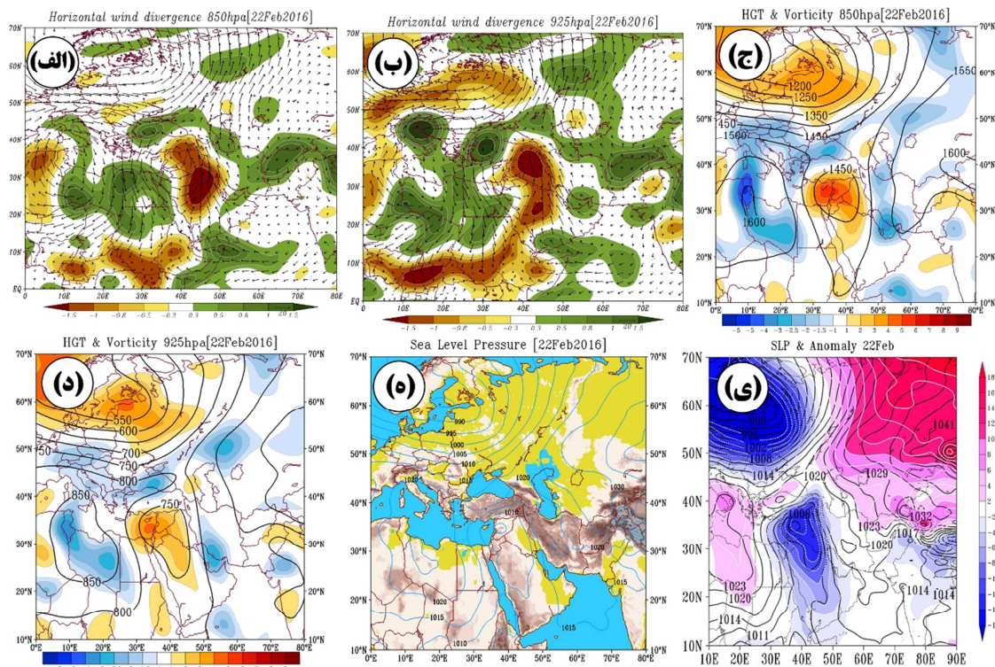
شکل ۶: نقشه‌های ترکیبی روز ۲۲ فوریه ۲۰۱۶؛ (الف) واگرایی افقی باد تراز ۸۵۰ ه.پ؛ (ب) واگرایی افقی باد تراز ۹۲۵ ه.پ؛ (ج) نقشه ترکیبی ژئوپتانسیل و تاوایی تراز ۸۵۰ ه.پ؛ (د) نقشه ترکیبی ژئوپتانسیل و تاوایی تراز ۹۲۵ ه.پ؛ (ه) نقشه فشار تراز دریا؛ (ی) نقشه ترکیبی فشار تراز دریا و آنومالی آن.
