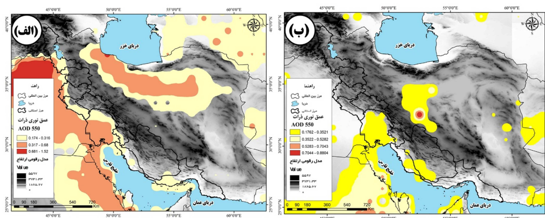
شکل ۴: توزیع فضایی عمق نوری ذرات (AOD550): (الف) ۲۱ فوریه ۲۰۱۶ میلادی و (ب) ۲۴ فوریه ۲۰۱۶ میلادی
