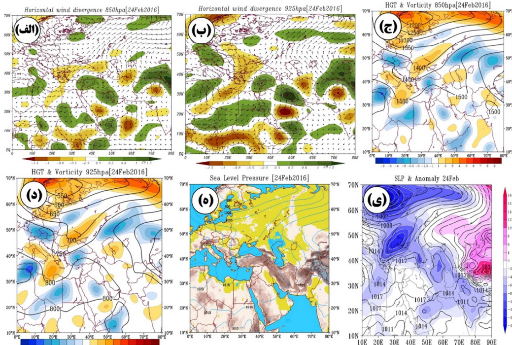
شکل ۸: نقشه‌های ترکیبی روز ۲۴ فوریه ۲۰۱۶: (الف) واگرایی افقی باد تراز ۸۵۰ ه.پ؛ (ب) واگرایی افقی باد تراز ۹۲۵ ه.پ؛ (ج) نقشه ترکیبی ژئوپتانسیل و تاوایی تراز ۸۵۰ ه.پ؛ (د) نقشه ترکیبی ژئوپتانسیل و تاوایی تراز ۹۲۵ ه.پ؛ (ه) نقشه فشار تراز دریا؛ (ی) نقشه ترکیبی فشار تراز دریا و آنومالی آن.
