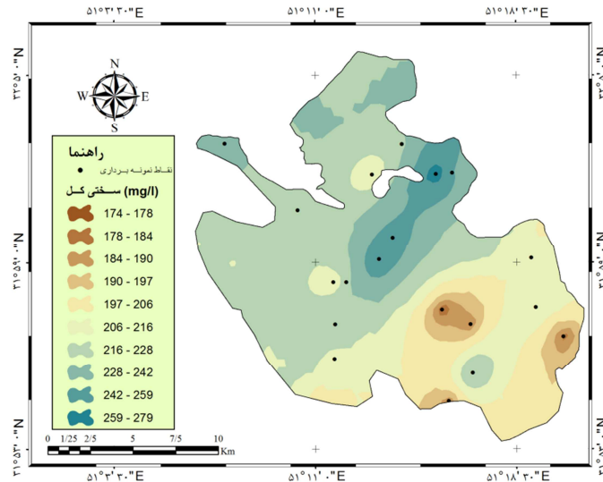
شکل ۳: نقشه تغییرات TH آب زیرزمینی دشت بروجن
