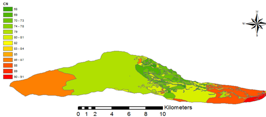
شکل ۷: نقشه شماره منحنی حوضه آبریز عموقین سال ۲۰۰۰
