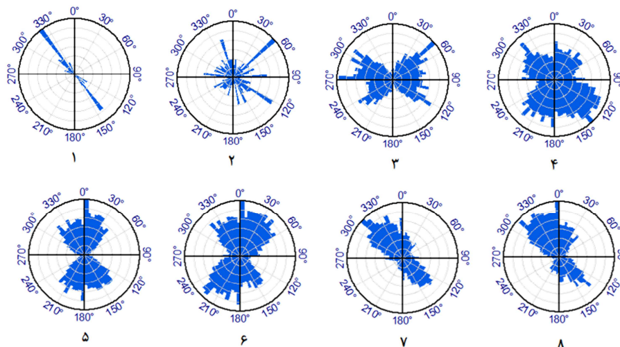
شکل ۲: نمودار رز خطواره‌ها: گسل‌ها ۱- به روش دستی، ۲- شبکه زهکشی، ۳- لندست ۸، ۴- تراسار ۱ x (HH)، ۵- سنتینل ۱ ۲ بالاگذر، ۶- سنتینل ۱ پایین گذر، ۷- الوس پالسا (HV)، ۸- الوس پالسا (HH)
