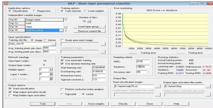
شکل ۱۳: ساختار شبکه عصبی برای ارزیابی آسیب پذیری در نرم افزار TerrSet.
