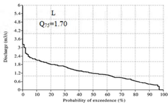
شکل ۴: منحنی دوام جریان ماهانه روخانه نساء (A) مهر، (B) آبان، (C) آذر، (D) دی، (E) بهمن، (F) اسفند (G) فروردین، (H) (I) خرداد، (J) تیر، (K) مرداد، (L) شهریور.
