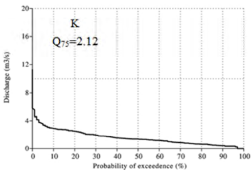
شکل ۴: منحنی دوام جریان ماهانه روخانه نساء (A) مهر، (B) آبان، (C) آذر، (D) دی، (E) بهمن، (F) اسفند (G) فروردین، (H) (I) خرداد، (J) تیر، (K) مرداد، (L) شهریور.
