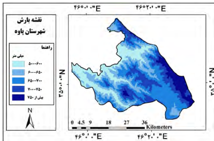
شکل ۲: نقشه بارش شهرستان پاوه.
