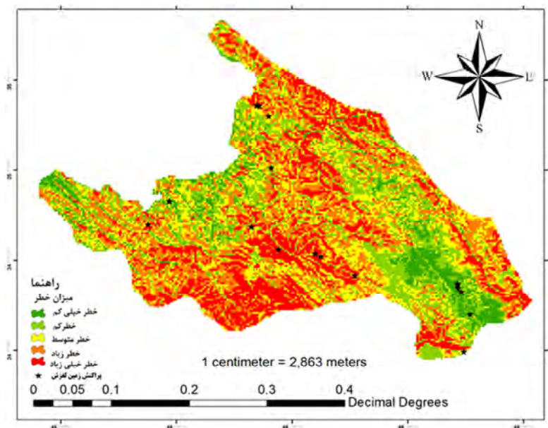
شکل ۸: نقشه پهنه‌بندی زمین‌لغزش شهرستان پابوه با استفاده از روش ANN.
