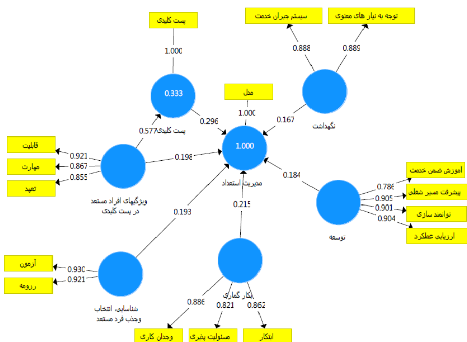
نمودار ۱. بارهای عاملی هر عامل خرده مقیاس در تحلیل معادلات ساختاری
