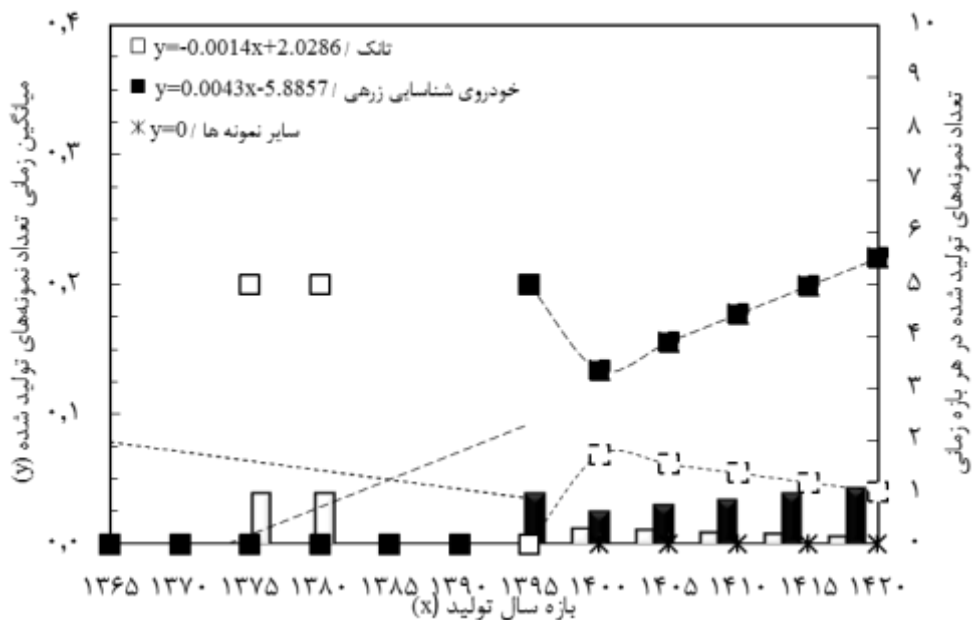
شکل (۲۱) نمودار میانگین زمانی تعداد نمونه‌های مختلف ادوات و تجهیزات خودروبی تولید شده در چشم‌انداز ارتقاء و بروزرسانی سیستم گلوله گذار خودرو و افزایش ایمنی خدمه آن
