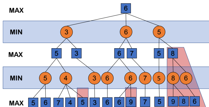
شکل (۷) نوع کارکرد روش هرس آلفا-بتا در کمینه بیشینه (Kopeck, 2016)
