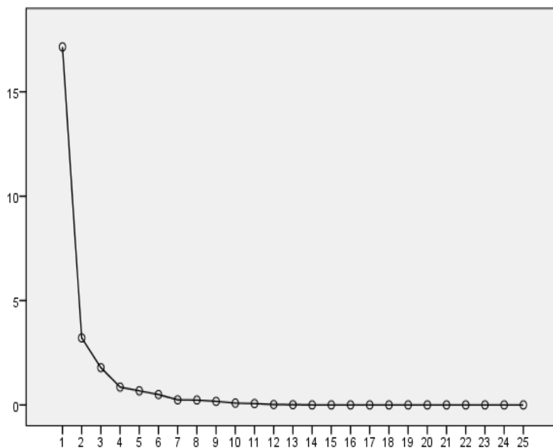
شکل (۱): نمودار اسکری کتل مؤلفه‌های استخراجی پرسشنامه
