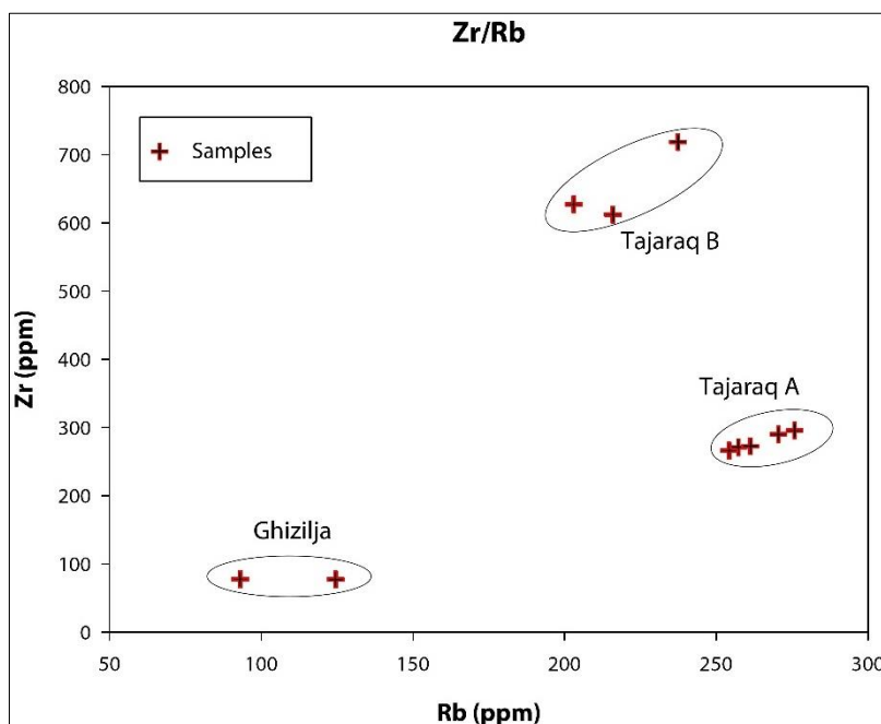
شکل ۸: نمودار پراکندگی زیر کونیوم به روییدوم (Zr/Rb) نمونه‌های آنالیز شده
