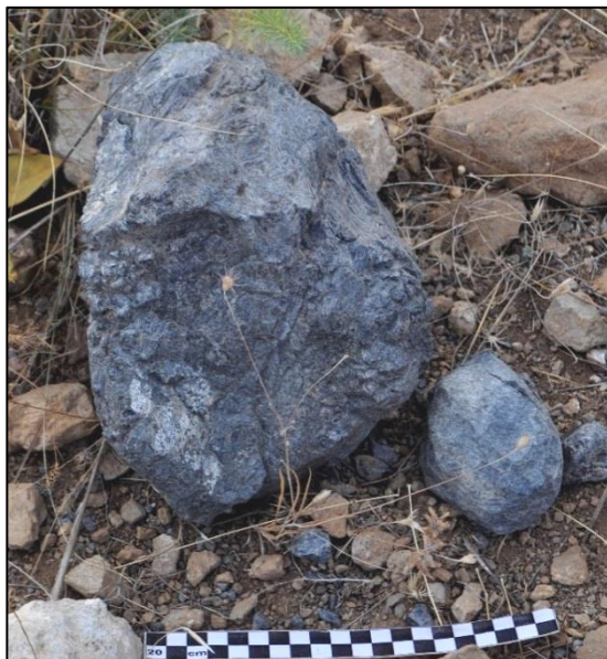
شکل ۶: نمای نزدیک از از واحد خرد شده حاوی ابسیدین در تجرق (دید به سمت جنوب) Fig. 6: A mesoscopic view of the crushed Obsidian particles at Tajaraq (view to South)
