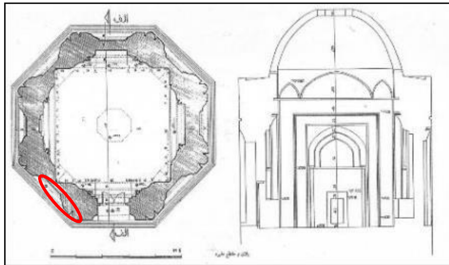
شکل ۲۰. پلان و مقطع مقبره خواجه اتابک، رنگ قرمز مربوط به محل کاشی‌های تراش خورده در نمای بناست [54]
