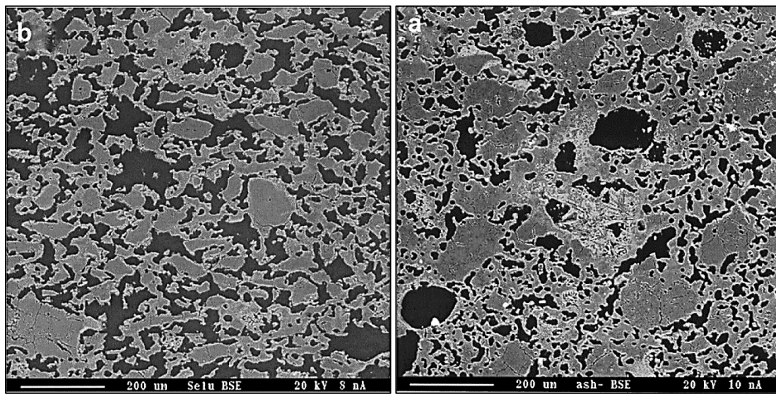
شکل ۱۷. تصویر SEM از بدنه نمونه سفال سلجوقی ایران؛ پیوستگی شبکه ذرات کوآرتز (خاکستری تیره) با ذرات شیشه پوششی ایجاد شده است [23].
