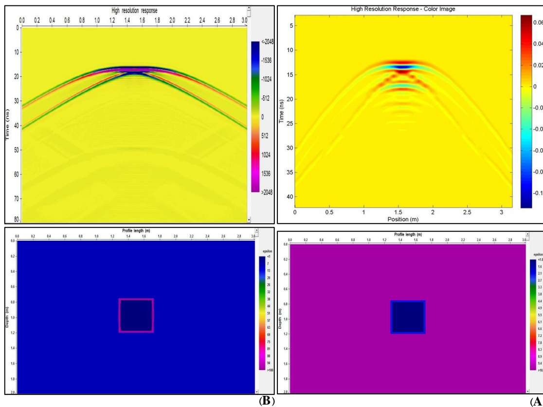
شکل ۹: مدل هندسی- فیزیکی - فیزیکی (هدایت الکتریکی در قسمت پایین) و پاسخ GPR آن (در قسمت بالا) برای تابوت با دو جنس مختلف (الف) چوبی و (ب) فلزی با پیمایش در راستای عمود بر امتداد طولی تابوت
