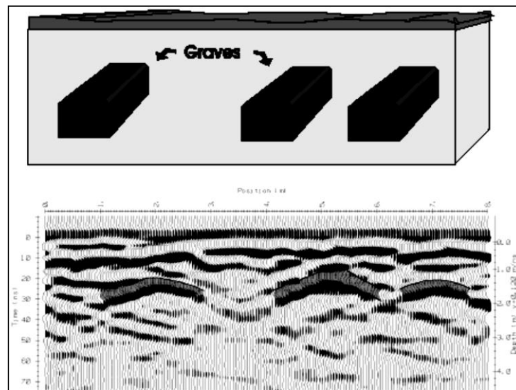
شکل ۶: شکل طرح وار سه قبر همراه با پاسخ سیستم GPR مربوطه [1] Fig. 6: Schematic picture of 3 graves with the related GPR system response [1]
