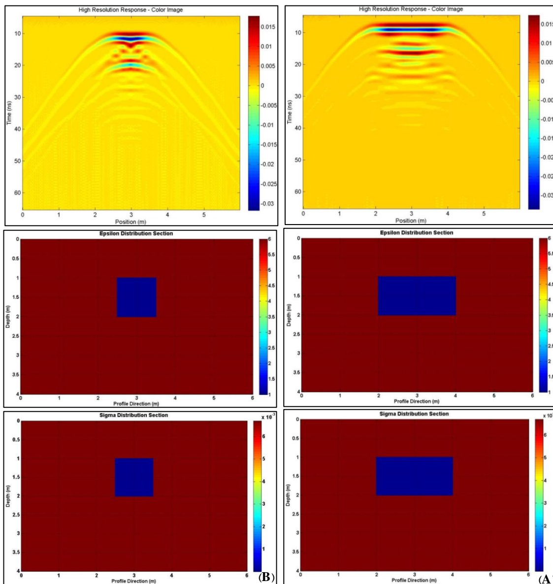
شکل ۷: مدل هندسی - فیزیکی (ردیف وسط، گذردهی دی‌الکتریک و ردیف پایین، هدایت الکتریکی) و پاسخ GPR آن (در قسمت بالا) برای (الف) پیمایش در راستای امتداد طولی یک قبر خالی و (ب) پیمایش در راستای عمود بر امتداد طولی یک قبر خالی
