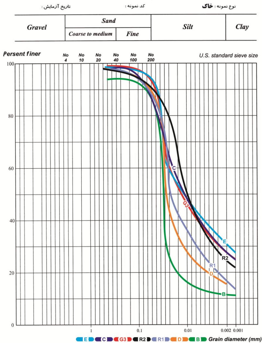
شکل ۲: دانه‌بندی به روش الک و هیدرومتری برای نمونه‌های مورد مطالعه [11]
