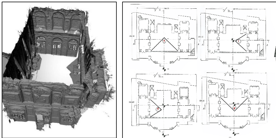
شکل ۷: یک دیوار به‌عنوان مبنا انتخاب‌شده و سایر دیوارها به دیوار مبنا اضافه‌شده، تالار اصلی ۴ نوبت اسکن شده است.
