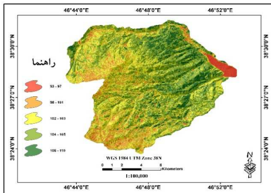
شکل ۱۱: نقشه تندی دامنه (شاخص توپوگرافی)
