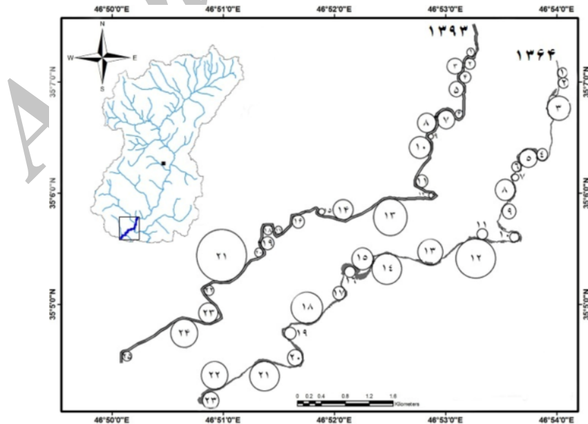
شکل ۵- دوایر مماس بر قوس‌های پیچان رودی بازه سوم در سال‌های ۱۳۶۴ و ۱۳۹۳
