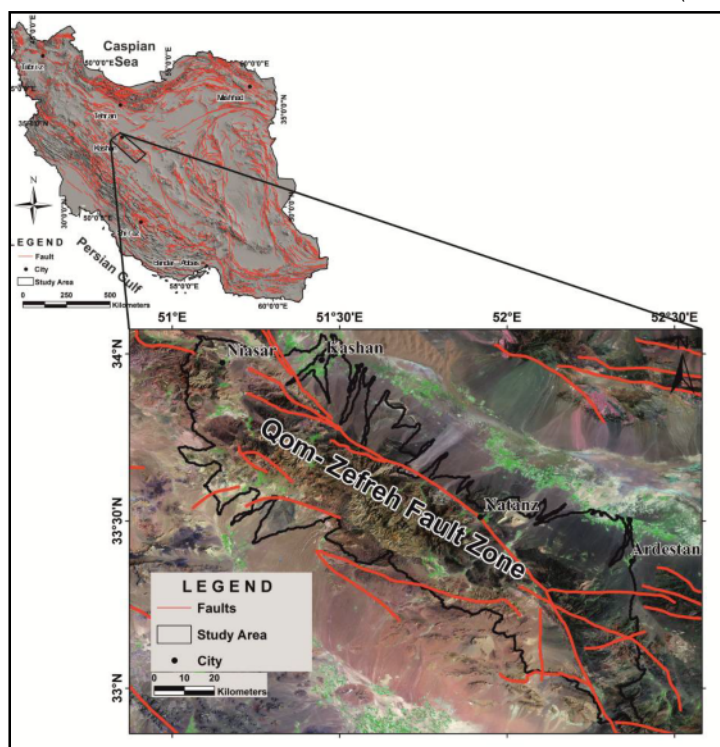
شکل ۱: منطقه مورد مطالعه در پهنه گسلی قم- زفره بر روی تصویر Mrsid
