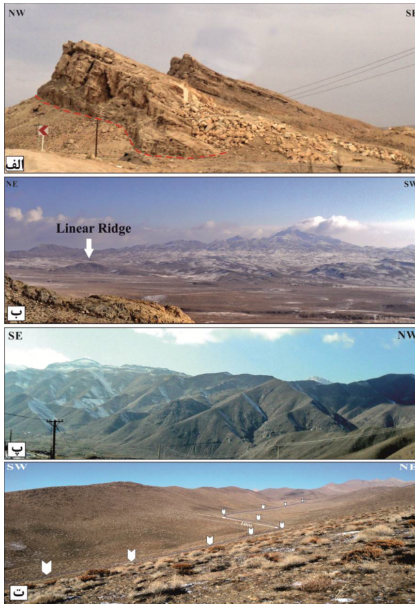
شکل ۱۸- شواهد لندفرهای مورفوتکتیکی فعال منطقه قم- زفره. الف) رانده شدن واحدهای الیگو میوسن بر روی کواترنر در پهنه گسلی قم- زفره، ب) نمونه‌ای از پشته‌های خطی در امتداد پهنه گسلی در منطقه مورد مطالعه، پ) سطوح مثلثی ایجاد شده در اثر فعالیت گسل قم- زفره، ت) نمونه‌ای از انحراف مسیر آبراهه ناشی از تأثیر فعالیت عهد حاضر گسل قم- زفره بر منطقه مورد مطالعه
