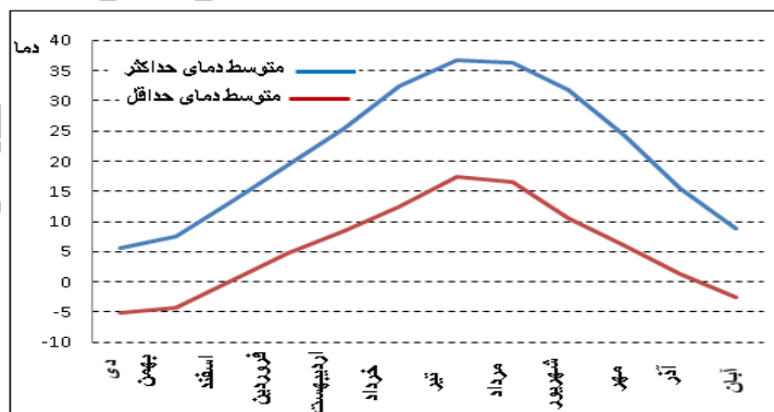
شکل ۷: متوسط دمای ماهیانه (درجه سانتی‌گراد) ایستگاه سنندج (۱۹۶۰-۲۰۰۵)
