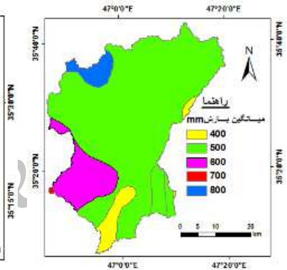
شکل ۶: نقشه متوسط بارندگی سالانه حوضه
