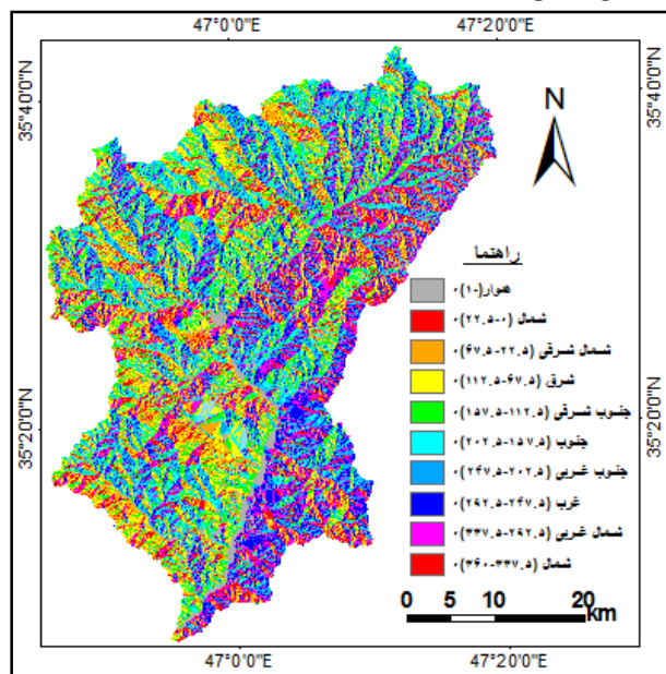
شکل ۱۳: نقشه جهت شیب حوضه قشلاق جدول ۳: توزیع سطوح جهت شیب حوضه قشلاق
