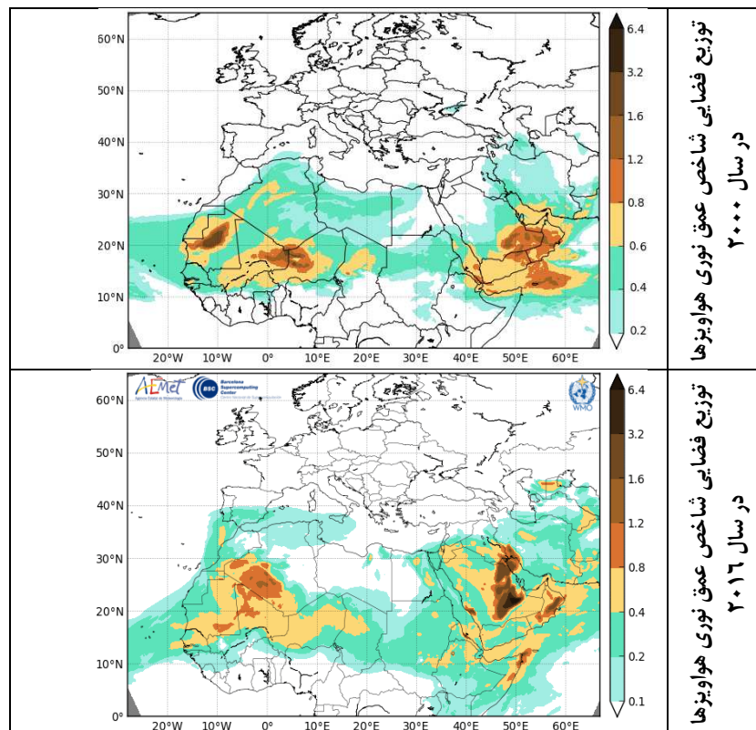
شکل ۸. توزیع فضایی شاخص عمق نوری آئروسول‌ها برای دو دوره ۲۰۱۶ و ۲۰۰۰ (میانگین دو ماه ژوئیه و اگوست) سازمان هواشناسی جهانی (WMO)
