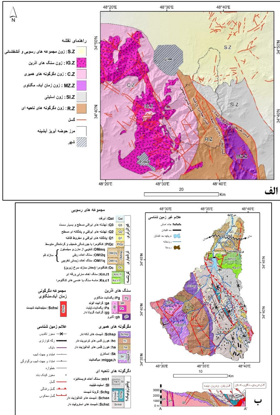
شکل ۲: الف) نقشه ساختمانی حوضه آبخیز آبشینه و اطراف ب) نقشه زمین شناسی حوضه آبخیز مورد مطالعه.
