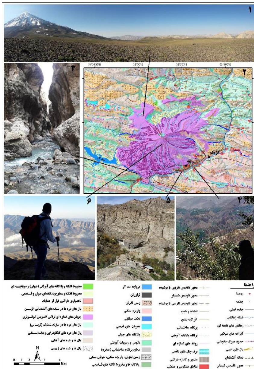
شکل ۹: ژئومورفولوژی منطقه مورد مطالعه: (۱) دشت سرداغ و دماوند، (۲) نقشه ژئومورفولوژی، (۳) تنگ تارپون، (۴) پادگانه‌های روستای نیاک، (۵) تراورتن آبسک و دخمه‌های سنگی کافر کلی، (۶) نمایی از دره هراز در ارتفاع ۴۶۰۰ متری قله دماوند
