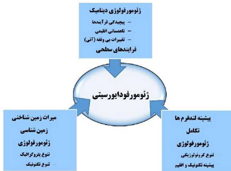
شکل ۱: اجزای ژئومورفودایورسیتی (توماس، ۲۰۱۲)
