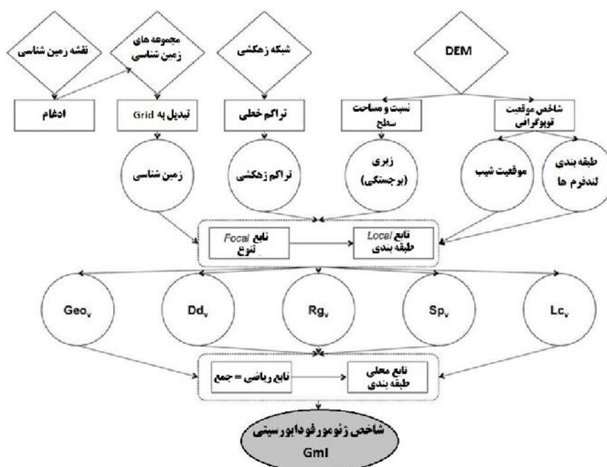
شکل ۳: مراحل اجرای شاخص ژئومورفودایورسیته (ملهلی و همکاران، ۲۰۱۷)
