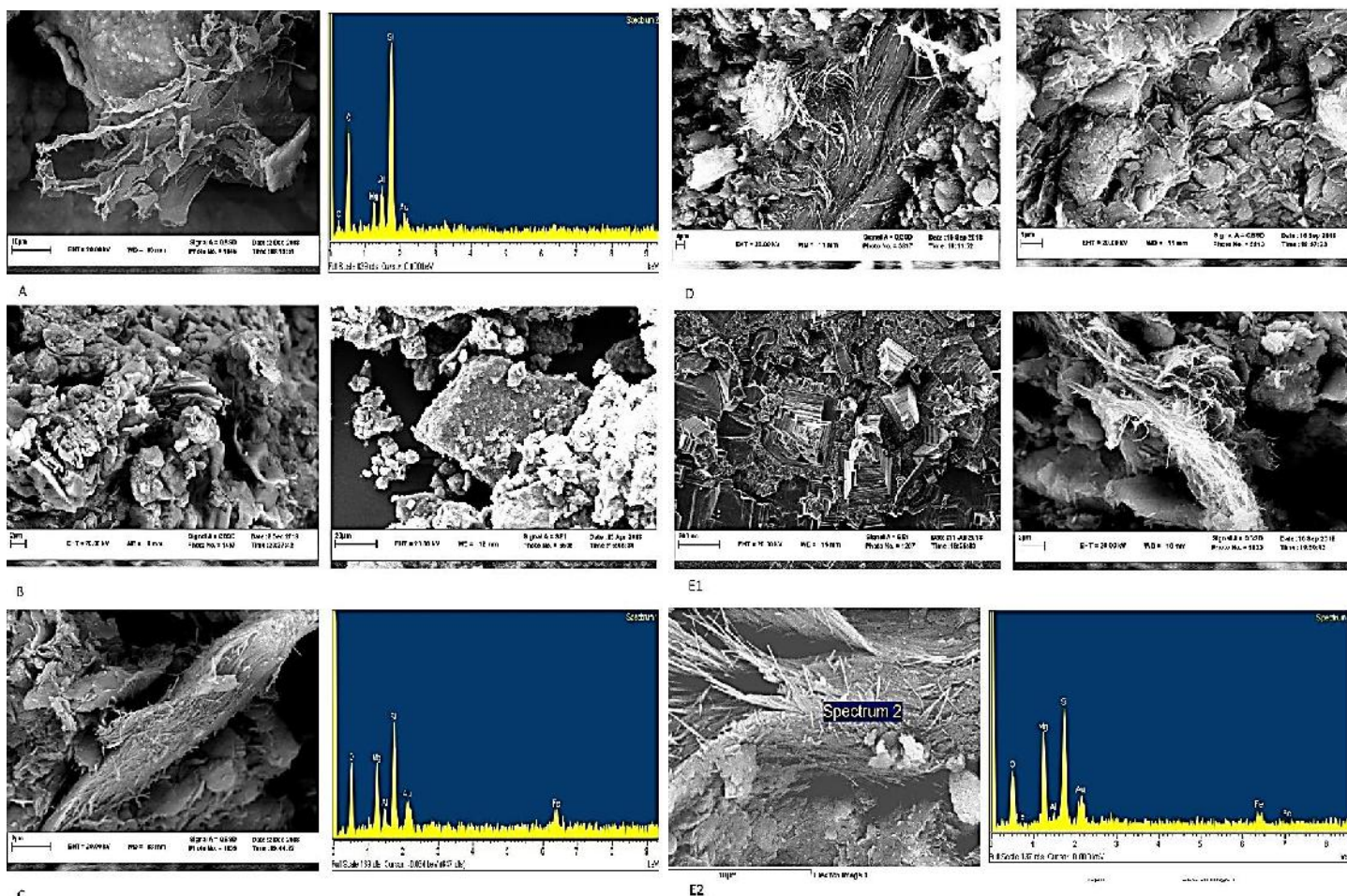
شکل ۶: تصویر ریزنگاشت میکروسکوپ الکترونی روبشی لایه‌های (A) کانی رسی اسمکتیت همراه با EDS آن در عمق ۳۰ سانتی متر (B) عدم وجود کانی رسی اتوزنیک در عمق ۱۰۰ (و ۷۰ سانتی متر (C) کانی رسی سپولیت در عمق ۳۰ سانتی متر (D) کانی رسی پالیگورسکیت در عمق ۱۰۰ سانتی متر (E1) وجود بلورهای کامل هالیت و کانی رسی پالیگورسکیت در عمق ۳۰ و ۷۰ سانتی متر (E2) کانی رسی سپولیت در عمق ۱۰۰ سانتی متر
