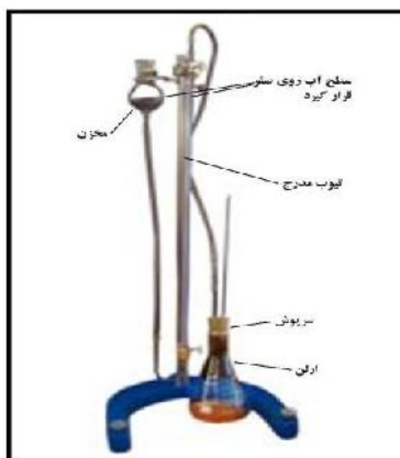
شکل ۱۱: دستگاه کلسیمتر برنارد
