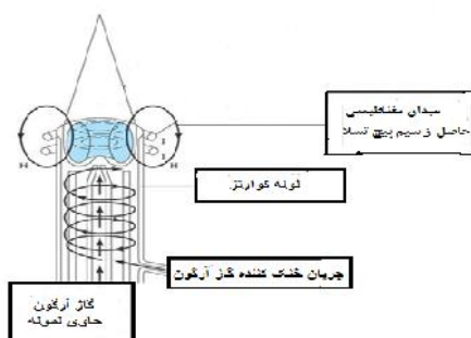
شکل ۱۲: نمایی از مشعل ICP و اجزاء جانبی آن
