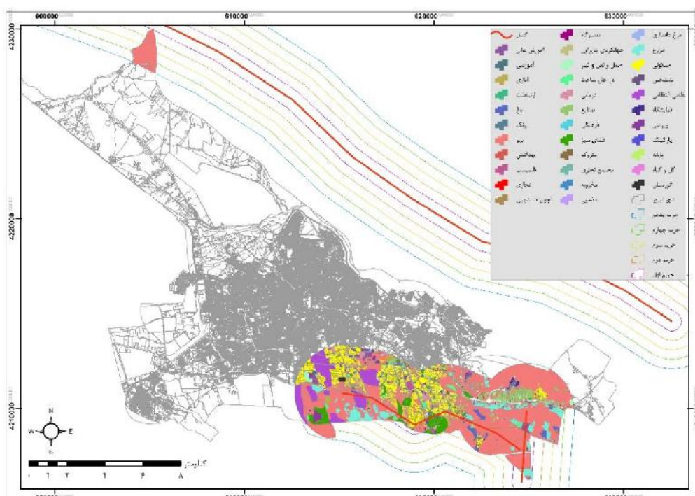
نقشه ۷: پراکنش کاربری‌های موجود در حریم گسل
