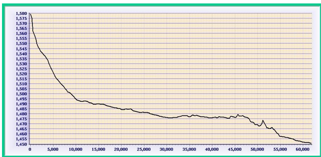
شکل ۲: نیمرخ طولی بازه مورد مطالعه رودخانه سیلاخور
