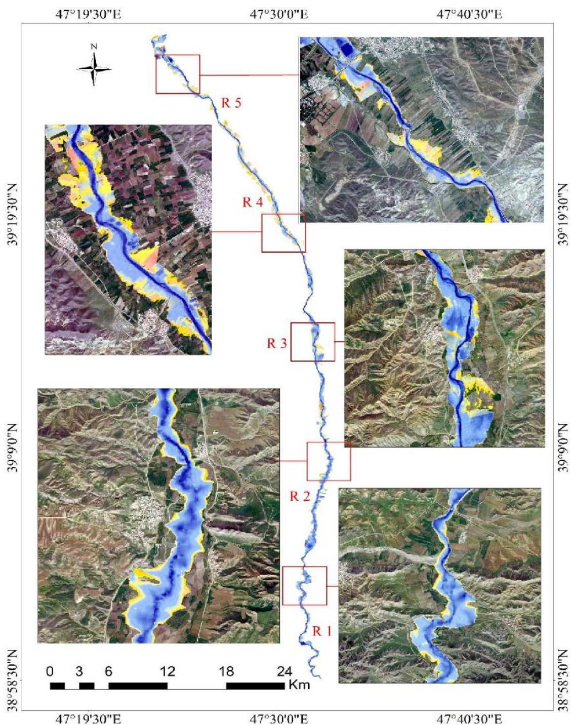
شکل ۴: شبیه‌سازی سیلاب‌های رودخانه دره انورت به تفکیک ۵ بازه مورد مطالعه
