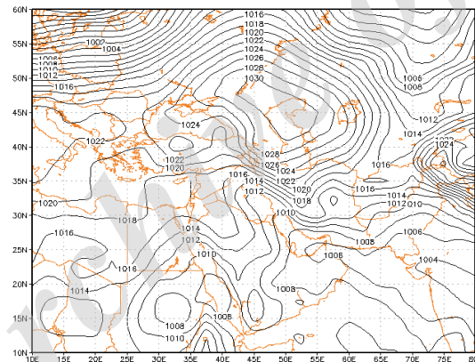
شکل ۵. نقشه فشار سطح زمین ۹ مهر ۱۳۸۰
