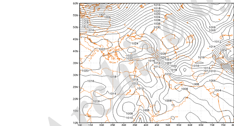
شکل ۵. نقشه فشار سطح زمین ۹ مهر ۱۳۸۰
