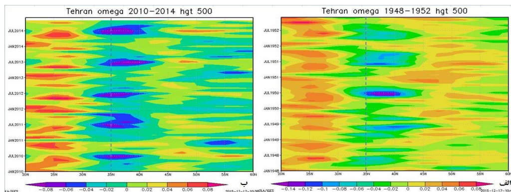
شکل ۵. محدوده‌ی زمانی استقرار شرایط صعودی و موقعیت تهران از آن در دو بازه: الف) در بازه‌ی ۵ ساله‌ی اول (۱۹۴۸-۱۹۵۲) و ب) در بازه‌ی ۵ ساله‌ی دوم (۲۰۱۰-۲۰۱۴). در بازه‌ی ۵ ساله دوم محدوده‌ی زمانی شرایط صعودی از بازه اول افزایش یافته است.
