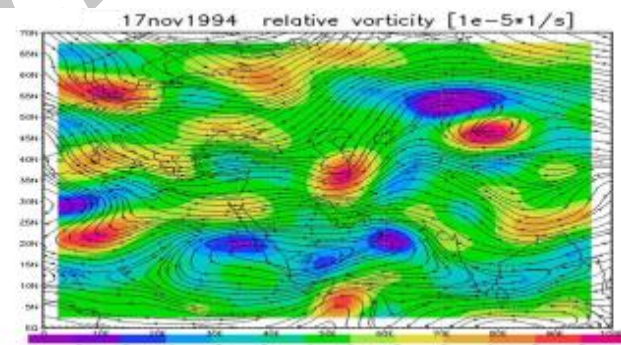
شکل ۲۴: نقشه تاوایی و خطوط جریان در تراز ۱۰۰۰ هکتوپاسکال در روز ۱۷ نوامبر ۱۹۹۴
