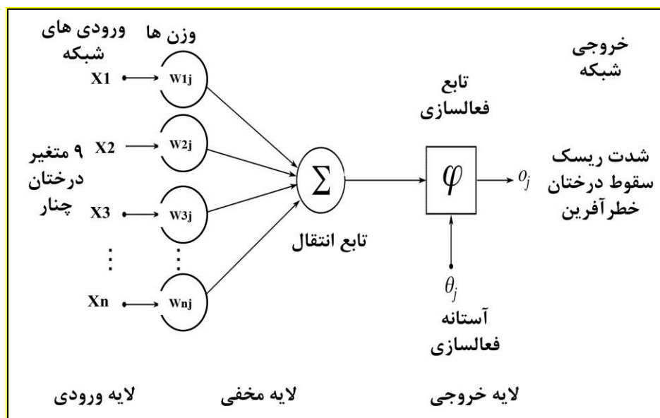
شکل ۱: شبکه پرسپترون با یک لایه مخفی
