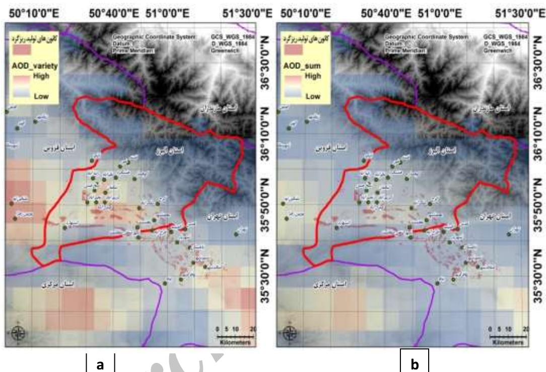
شکل ۶- نقشه ارزیابی صحت کانون‌های تولید ریزگرد به کمک تغییرات آماری عمق اپتیکی هواپز سال ۲۰۱۰ تا ۲۰۱۵ - اعتبارسنجی کانون‌های ریزگرد با استفاده از اطلاعات ایستگاه‌های پایش آلودگی هوا و سینوپتیک (کد ۰۶ و ۰۷)
