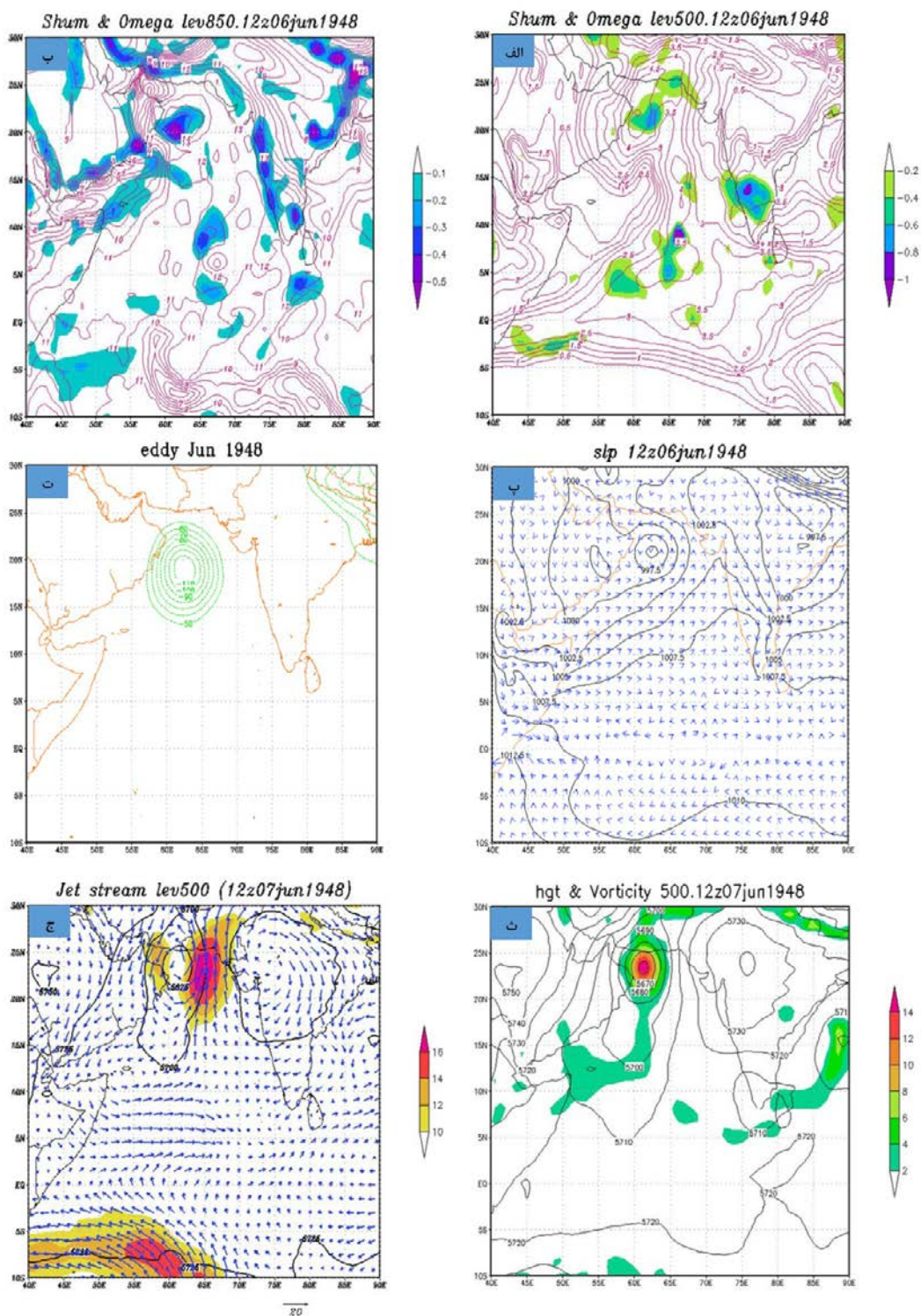
شکل ۴- الف تا ج به ترتیب نم و بیژه و سرعت قائم تراز ۵۰۰ میلی بار، نم و بیژه و سرعت قائم تراز ۸۵۰ میلی بار، فشار تراز دریا، پیچانه جوی تراز ۵۰۰ میلی بار (ساعت ۱۲ روز ۰۶ ژوئن ۱۹۴۸)، ارتفاع ژئوپتانسیل و فرارفت تاوایی تراز ۵۰۰ میلی بار و رودباد تراز ۵۰۰ میلی بار ساعت ۱۲ روز ۰۷ ژوئن ۱۹۴۸
