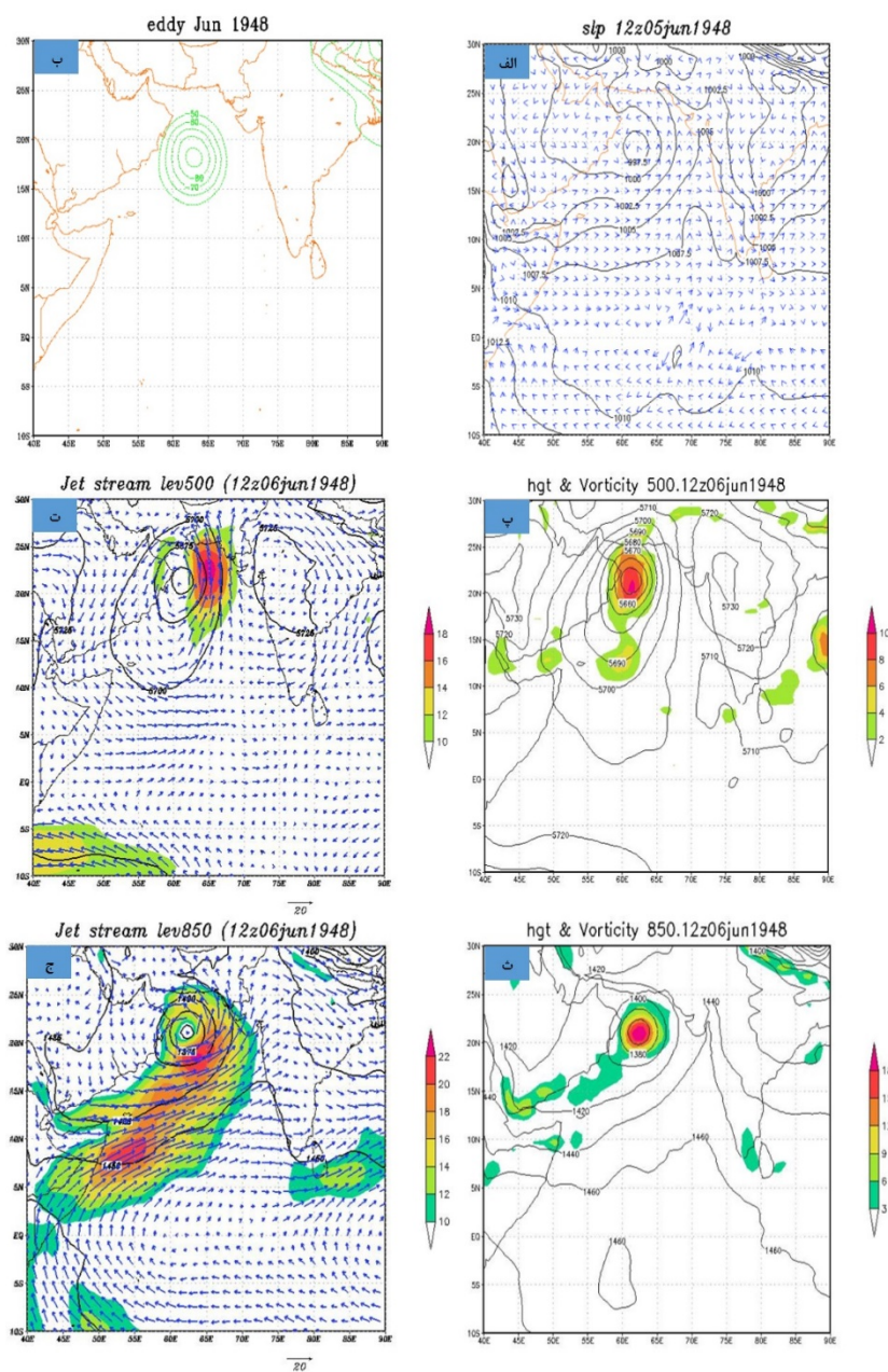
شکل ۳- الف تا ج به ترتیب فشار تراز دریا، بیجان جوی تراز ۵۰۰ میلی بار (ساعت ۱۲ روز ۰۵ ژوئن ۱۹۴۸)، ارتفاع ژئوپتانسیل و فرارفت تاوایی تراز ۵۰۰ میلی بار، رودباد تراز ۵۰۰ میلی بار، ارتفاع ژئوپتانسیل و فرارفت تاوایی تراز ۸۵۰ میلی بار و رودباد تراز ۸۵۰ میلی بار ساعت ۱۲ روز ۰۶ ژوئن ۱۹۴۸
