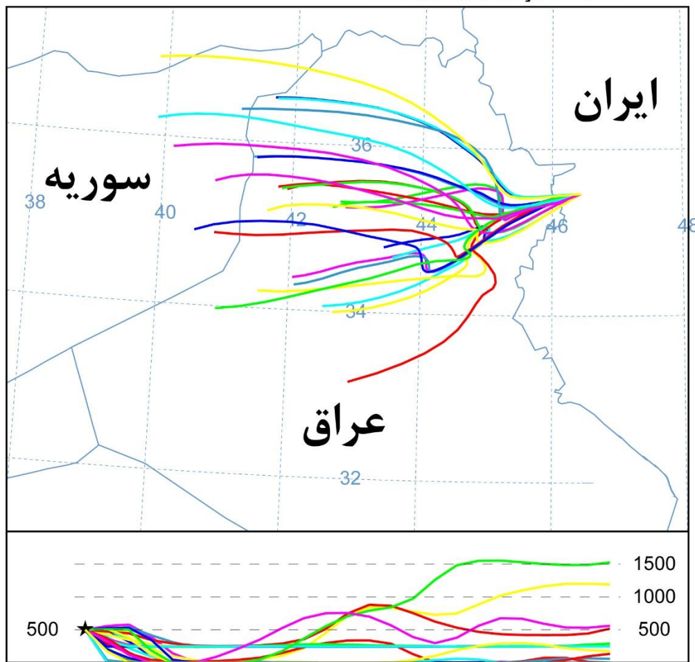
شکل ۸- ردیابی پسگرد مسیرهای گردوغبار با گام زمانی ۶ ساعته تا ۲۴ ساعت قبل از ورود اولین گرد و غبار
