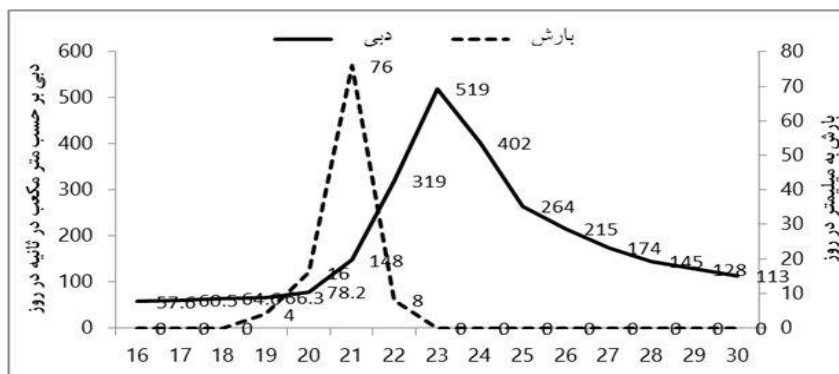
شکل ۲. آبنمود سیلاب اسفند ۱۳۸۳
