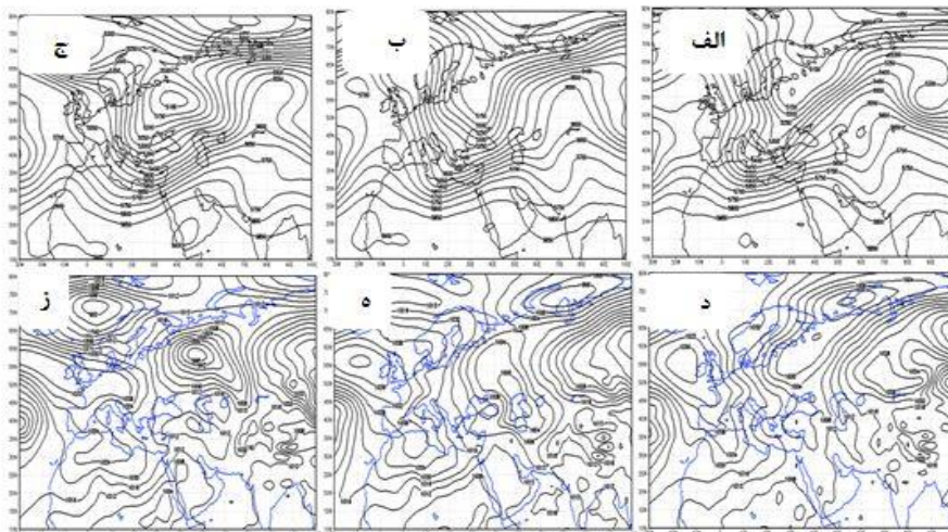
شکل ۳. نقشۀ ارتفاع ژئوپتانسیل و ارتفاع تراز دریا در روزهای هجدهم، نوزدهم و بیستم اسفند ۱۳۸۳ به ترتیب از راست به چپ
