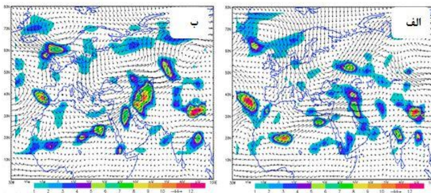
شکل ۴. نقشه شار رطوبتی روزهای نوزدهم و بیستم اسفند ۱۳۸۲ به ترتیب از راست به چپ
