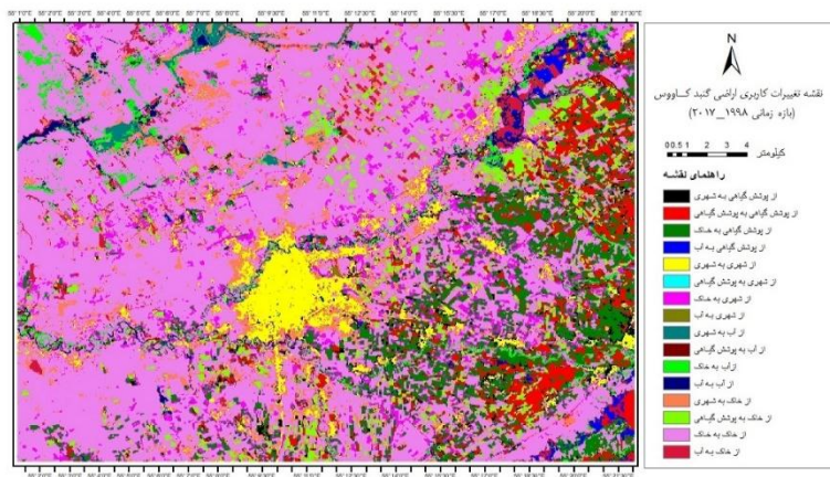
شکل ۶. نقشه تغییرات پوشش اراضی شهرستان گنبدکاووس برای سال‌های ۱۹۹۸-۲۰۱۷
