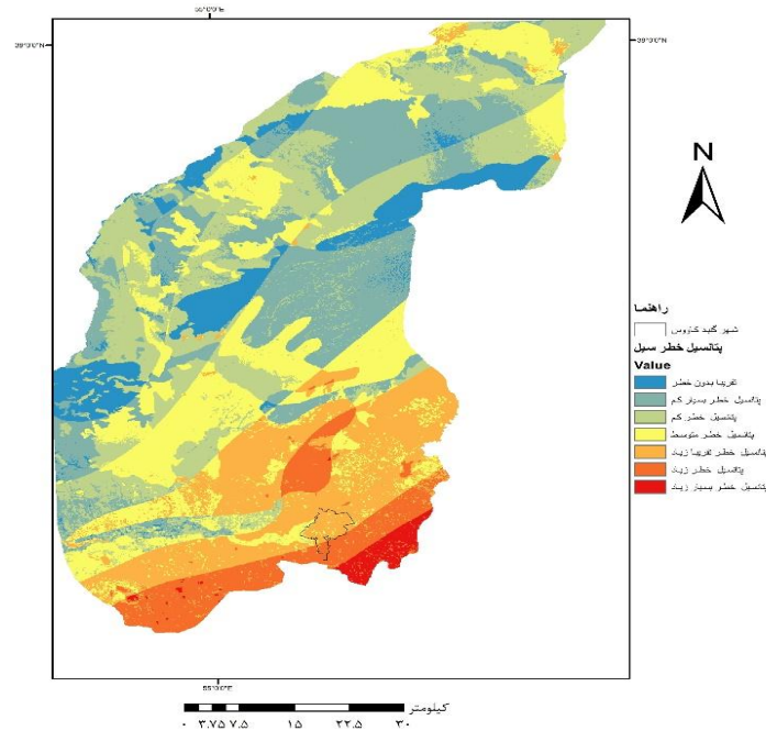
شکل ۴. نقشه رده‌بندی شده پتانسیل سیل خیزی گیلدکاوس
