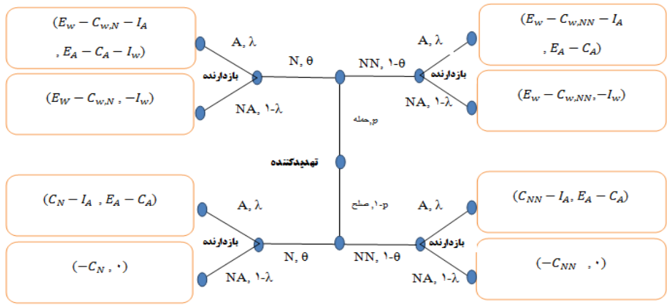
شکل (۲): گراف بازی پویای بازدارندگی با اطلاعات ناقص. بازیکن اول در حالت جنگ و صلح قرار دارد و در هر حالت می‌تواند با احتمال مشخصی علامت‌های هنجار (N) و ناهنجار (NN) از خود بروز دهد و بازیکن دوم در یک حالت در محیط قرار دارد و می‌تواند در مقابل راهبردهای تهدیدکننده اقدام (A) یا عدم اقدام (NA) را انتخاب نماید.
