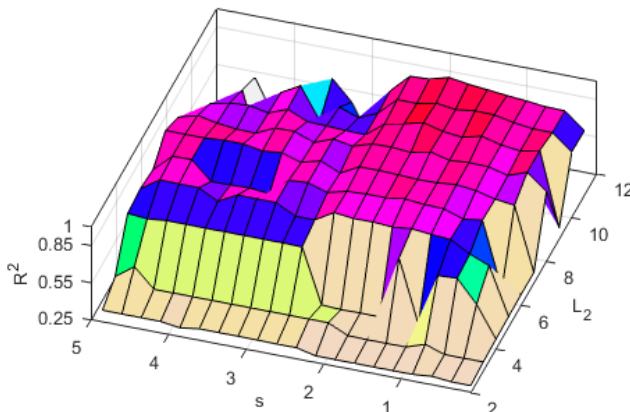
شکل ۲. تغییرات R^2 شبکه RBF بر حسب دو عامل تعداد نرون‌ها در لایه مخفی ( L_2 ) و مقادیر پارامتر گستردگی (s)
