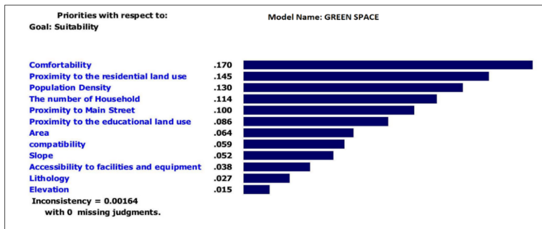
شکل ۴. بردار وزنی
